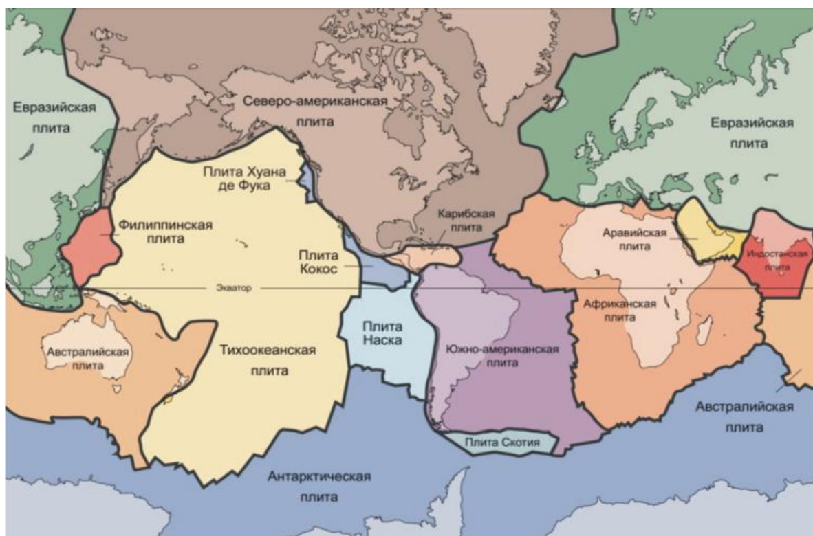
Рис.2. Литосферные плиты и современные материки.
