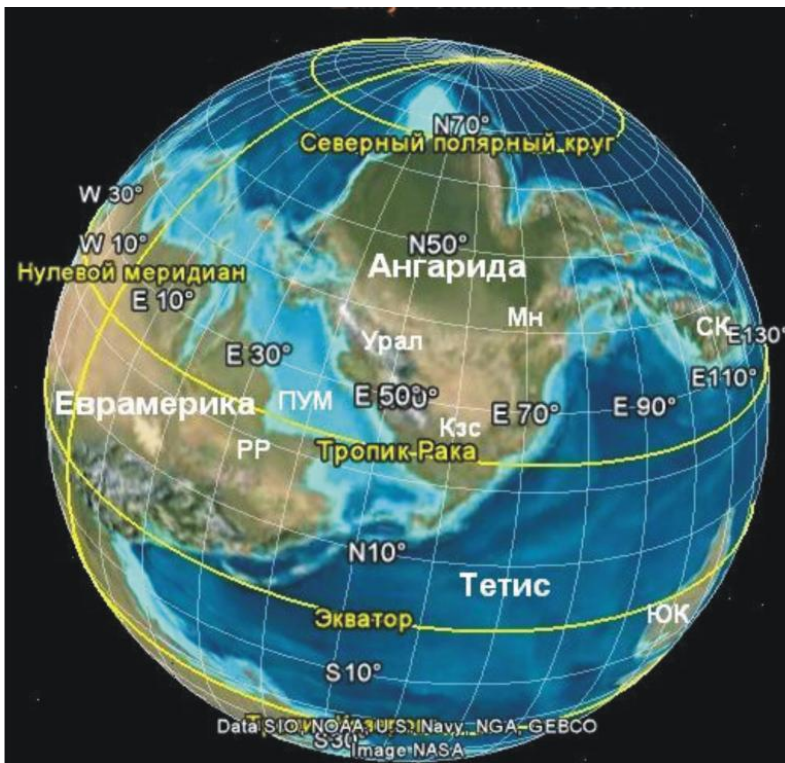
Рис.1. Ангарида как составная часть единого материка Пангеи.
