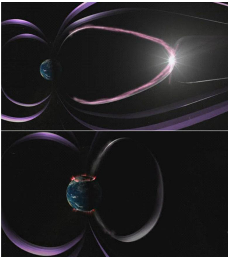
Рис.7. Поток высокоэнергетических частиц вытянутой области магнитного поля возвращается к Земле и проявляется в виде полярных сияний.
